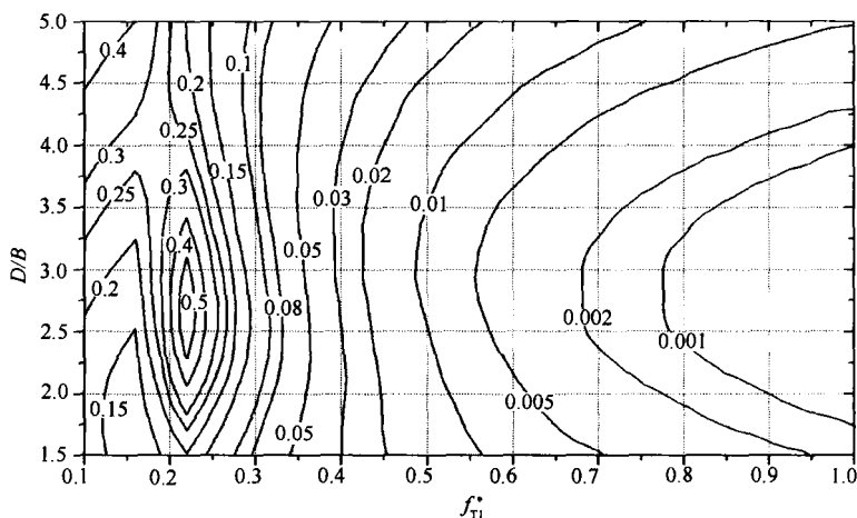
图 H. 3. 4 扭矩谱能量因子
