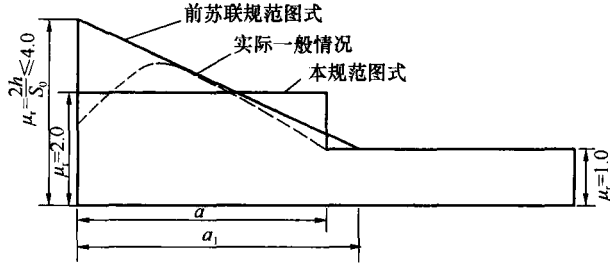
图 5 高低屋面处雪堆分布图示
