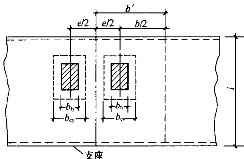
图 C.0.5-3 相邻两个局部荷载的有效分布宽度
