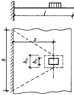
图 C. 0. 5-4 悬臂板上局部荷载的有效分布宽度
