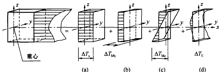
图 9 结构构件任意截面上的温度分布
