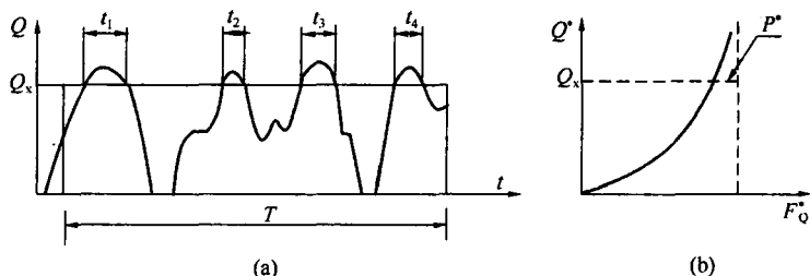
图 1 可变荷载按持续时间确定代表值示意图
