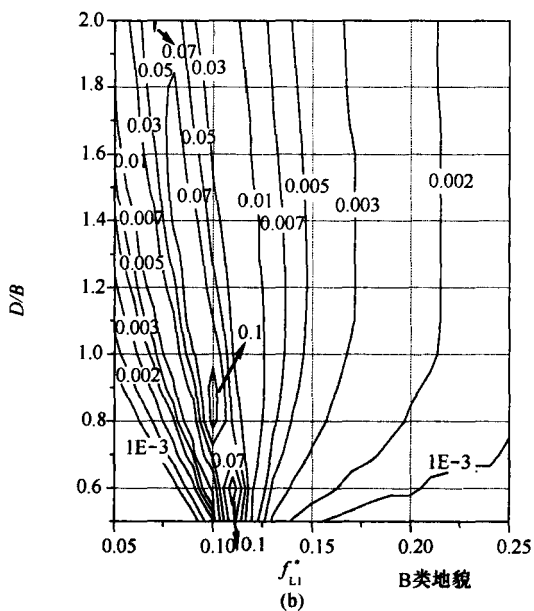
图 H.2.4 无量纲横风向广义风力功率谱 (一)
