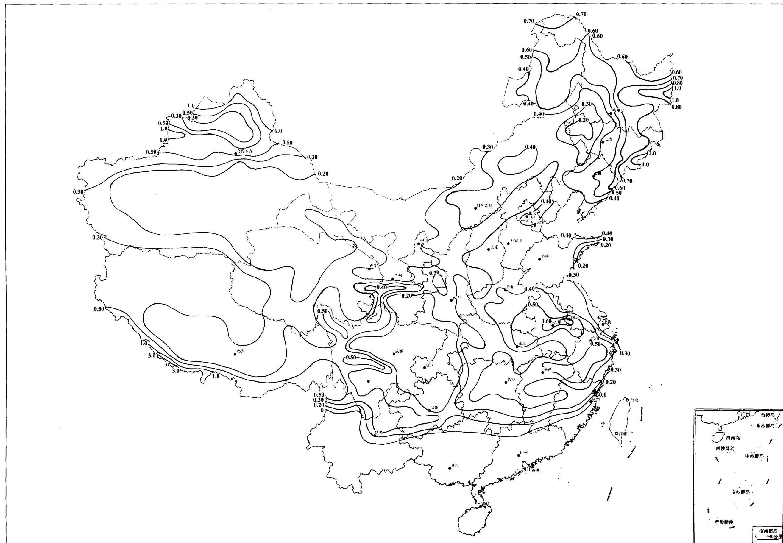
图 E. 6. 1 全国基本雪压分布图( \text{kN/m}^2 )
