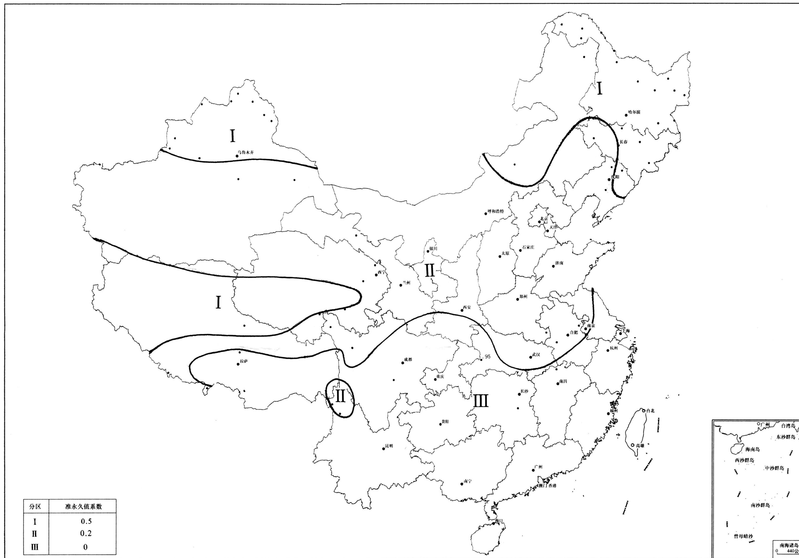
图 E. 6. 2 雪荷载准永久值系数分区图
