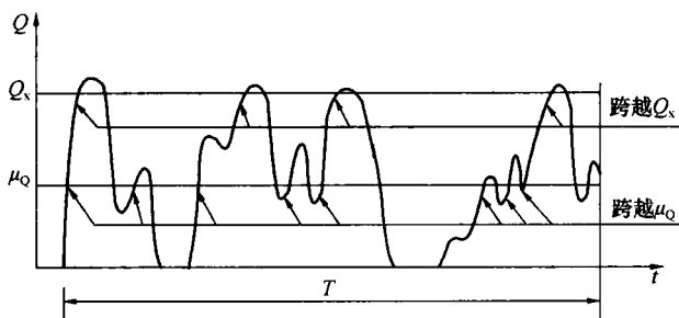
图 2 可变荷载按跨越率确定代表值示意图
