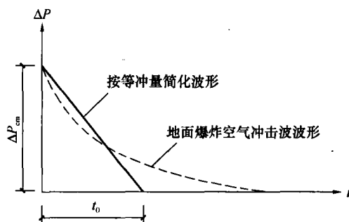
图 10 常规武器地面爆炸空气冲击波简化波形
