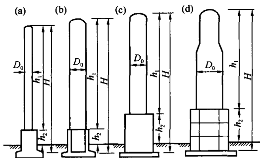
图 F.1.2 设备塔架的基础形式
