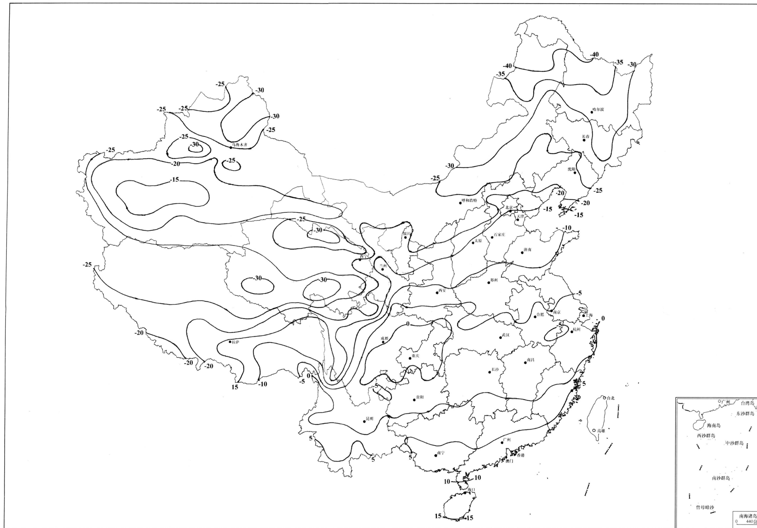
图 E. 6.5 全国基本气温(最低气温)分布图
