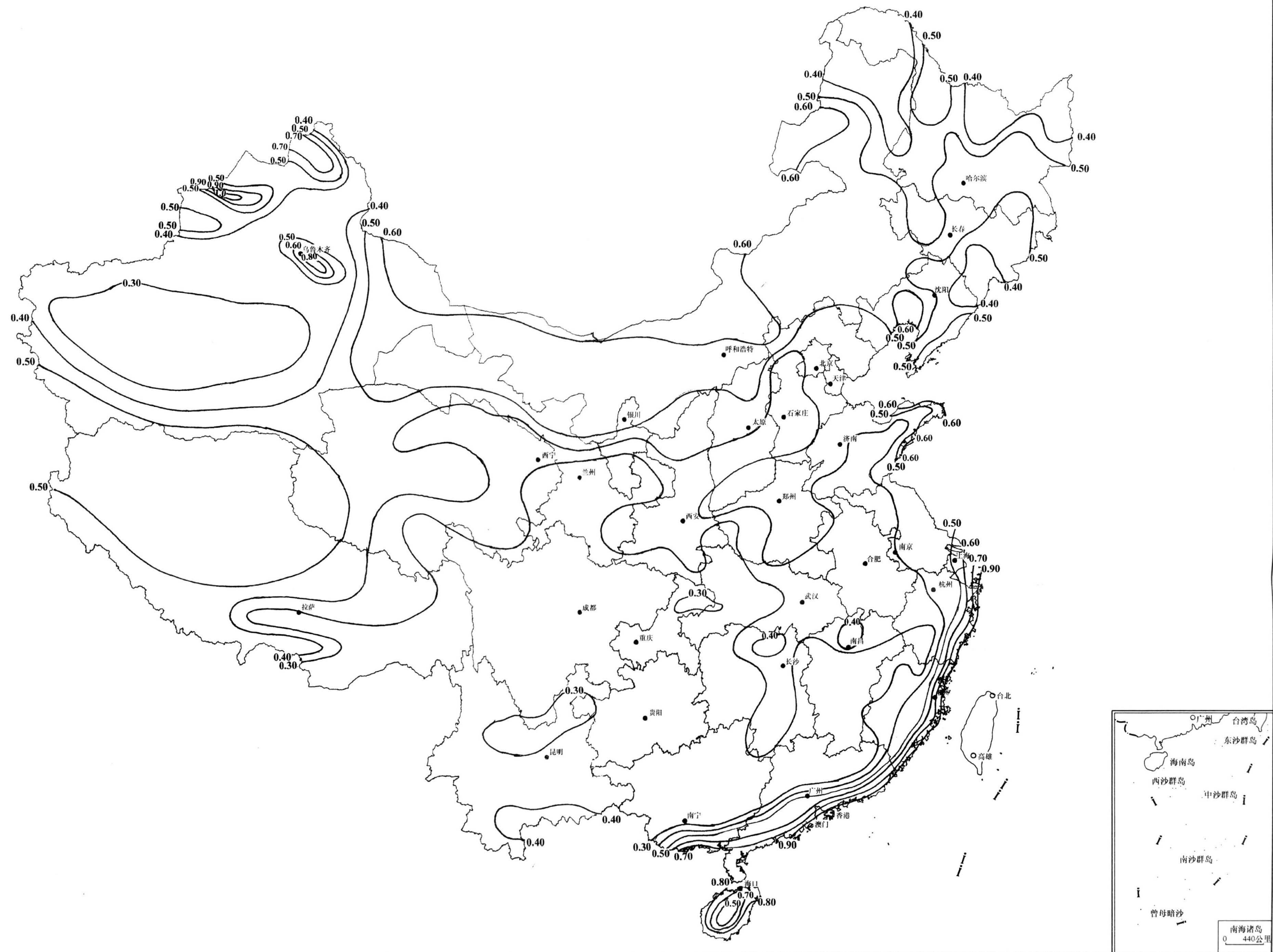
图 E. 6.3 全国基本风压分布图( \text{kN/m}^2 )
