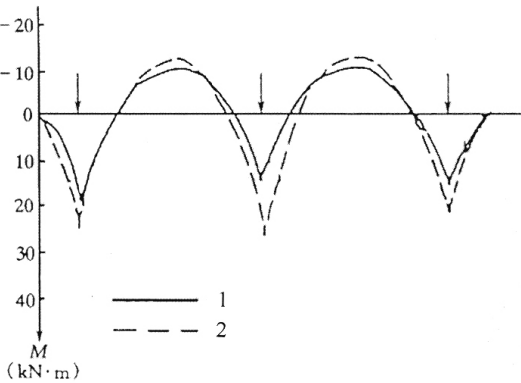
图 23 整体分析法与倒梁板法弯矩计算结果比较
