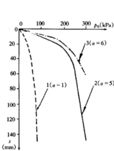
图 5 现场载荷试验 p-s 曲线
