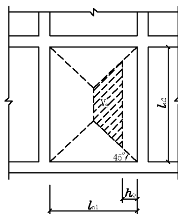
图 8.4.12-2 底板剪切计算示意
