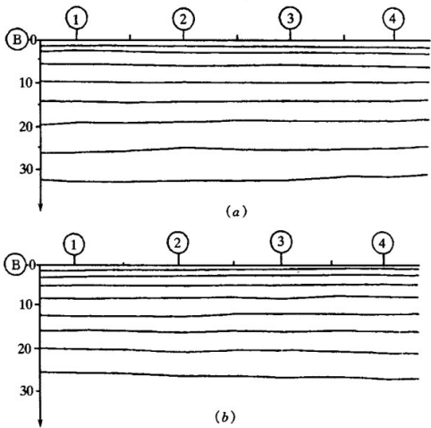
图 22 (B) 轴线沉降曲线
