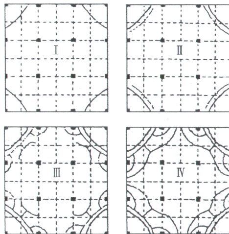
图 23 角柱（筒）下筏板验算剪切部位示意
