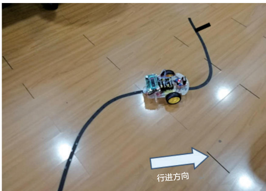
图4-17 循迹小车沿黑线运行图
