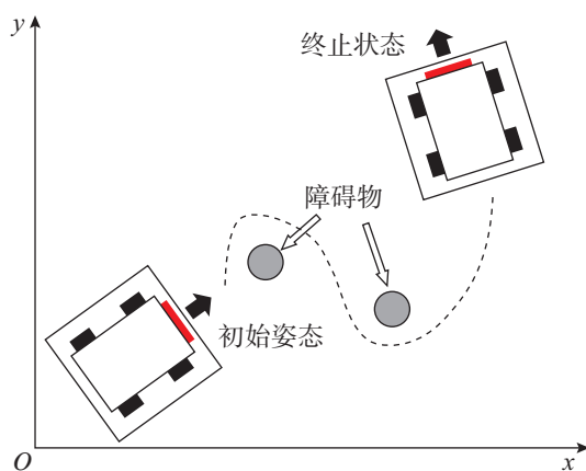
图4-5 移动机器人轨迹控制示意图
