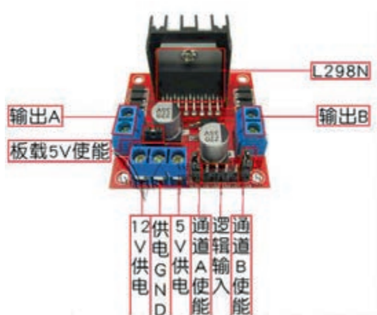
图 3-17 电机驱动模块
