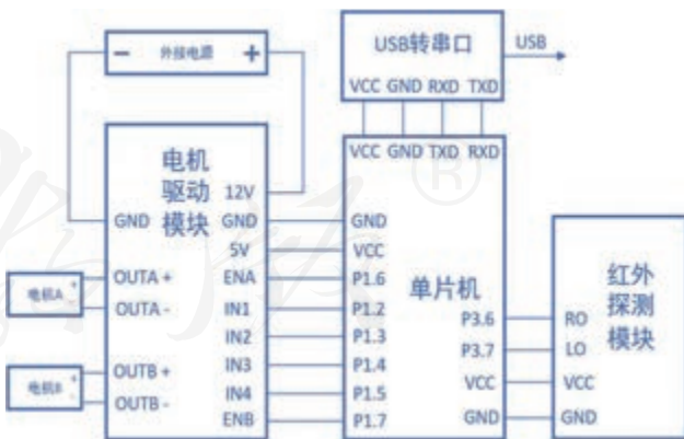
图 1-56 循迹小车电路图
