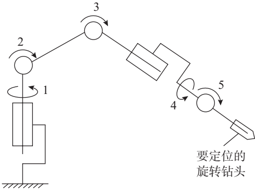
图1-38 使用机械臂对钻头进行定位定向
