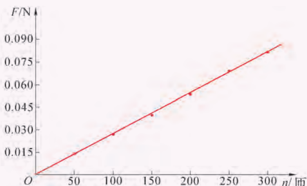
图 5-6 安培力与导线长度 (线圈匝数) 的关系
