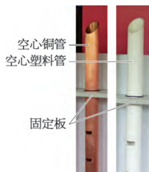
图 6-1 竖直放置的空心铜管和塑料管
