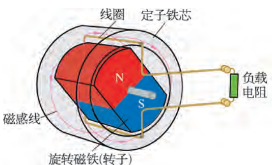
图 7-38 旋转磁极式发电机
