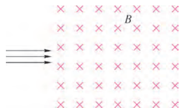
图 5-25 粒子束进入匀强磁场
