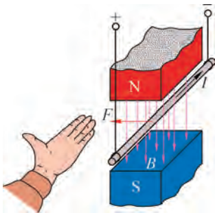
图 5-3 左手定则
