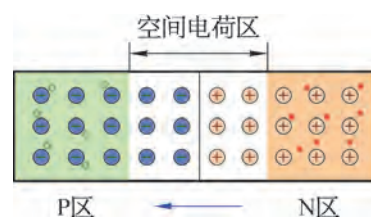
图 11-49 PN 结
