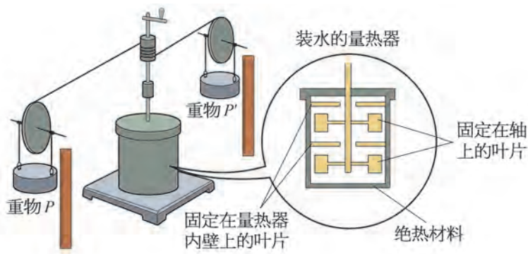
图 12-5 焦耳的实验装置
