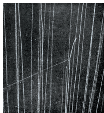
图 15-8 布拉凯特所摄的云室照片
