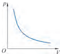
图 11-12 等温线
