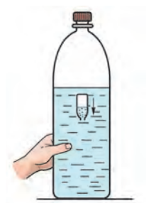
图 11-8 浮沉子
