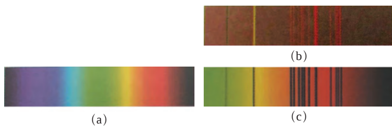
图 13-12 光谱
