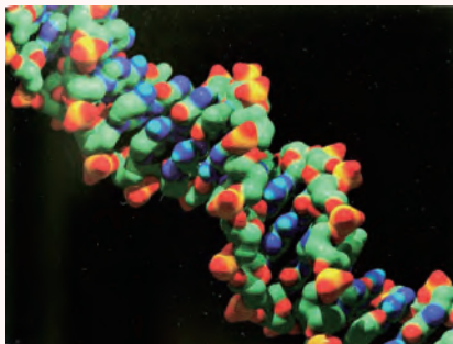
图 14-16 根据电子衍射实验推演的 DNA 大分子结构示意图
