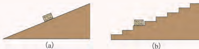
图 13-13 斜面 and 阶梯
