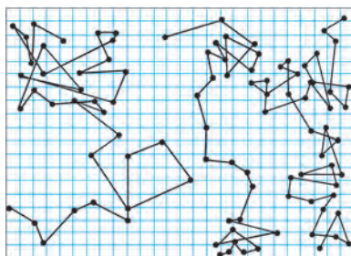
图 10-10 布朗运动
