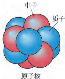
图 15-11 原子核模型
