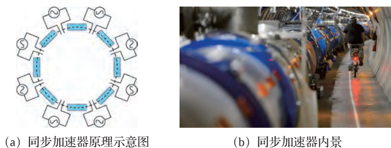
图 15-30 同步加速器
