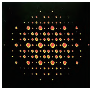
(a) 电子经单晶体衍射的图样
