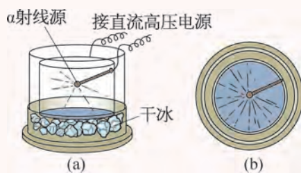
图 15-9 云室
