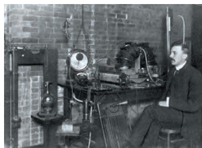
图 13-6 卢瑟福
