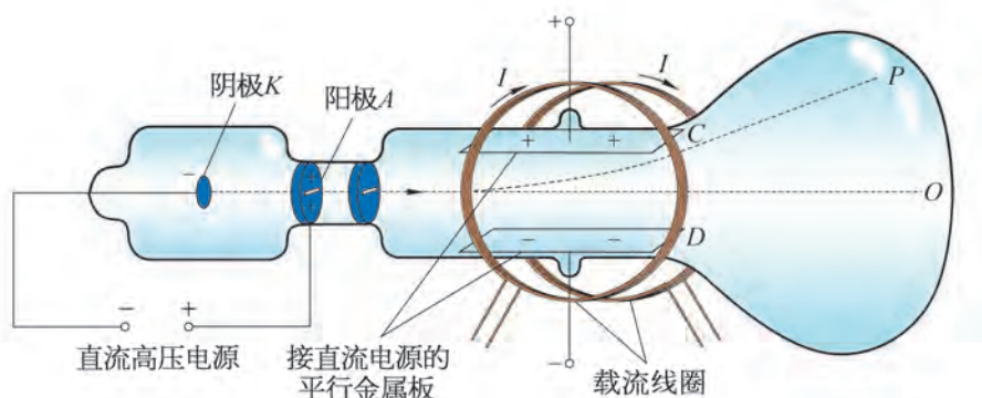
图 13-4 用静电偏转管测电子的比荷
