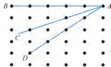
图 11-41 晶体各向异性的缘由
