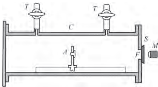
图 15-7 卢瑟福发现质子的实验装置示意图
