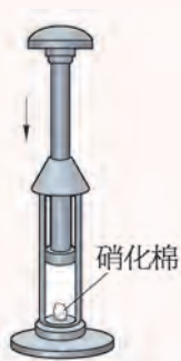
图 12-4 压缩气体做功，气体内能增加
