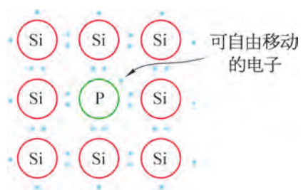
图 11-47 N 型半导体的共价键结构
