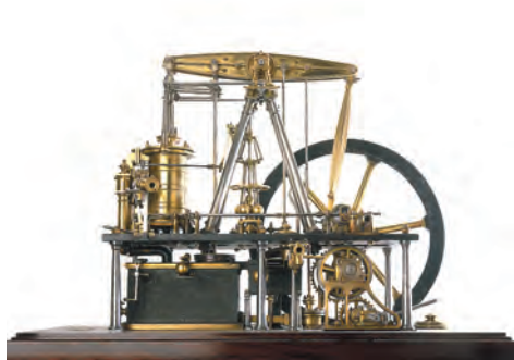
图 12-1 瓦特发明的高效率蒸汽机模型
