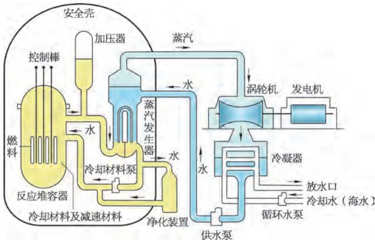
图 15-19 核电站示意图
