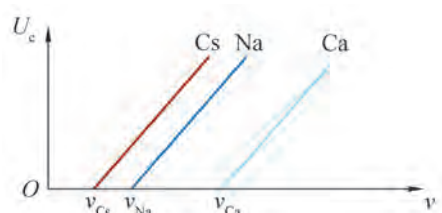
图 14-8 反向遏止电压 U_c 与入射光频率 \nu 的关系
