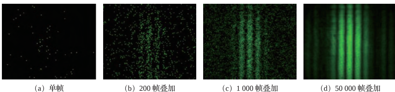
图 14-13 光子逐个通过双缝后的干涉图样
