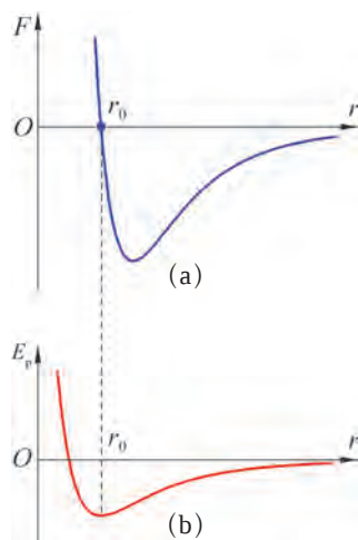
图 12-3 分子相互作用力和分子势能与分子间距离的关系
