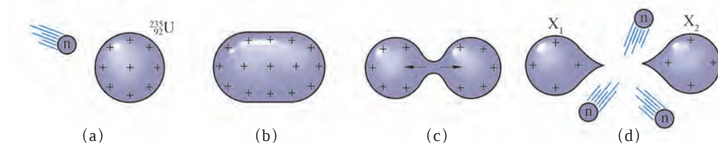
图 15-15 铀 235 裂变的液滴模型
