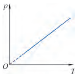
图 11-22 等容线
