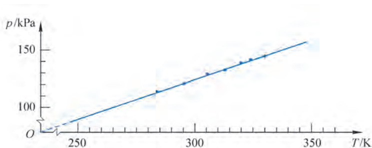
图 11-21 气体压强 p 与热力学温度 T 的关系
