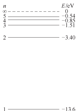
图 13-15 氢原子的能级图
