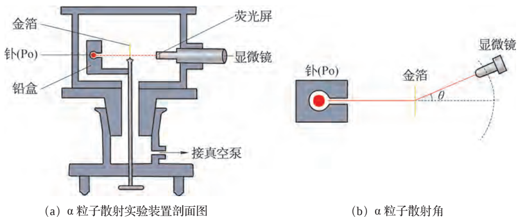
图 13-7 \alpha 粒子散射实验
