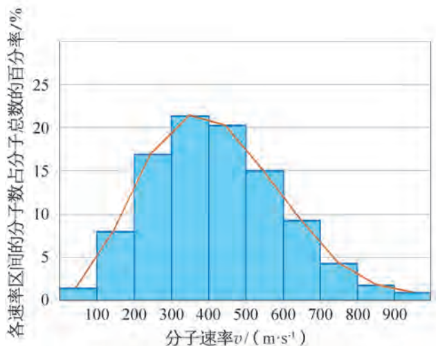
图 10-15 0℃时氧分子在各速率区间分布的直方图
