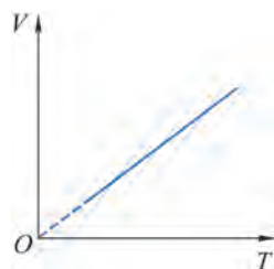
图 11-23 等压线
