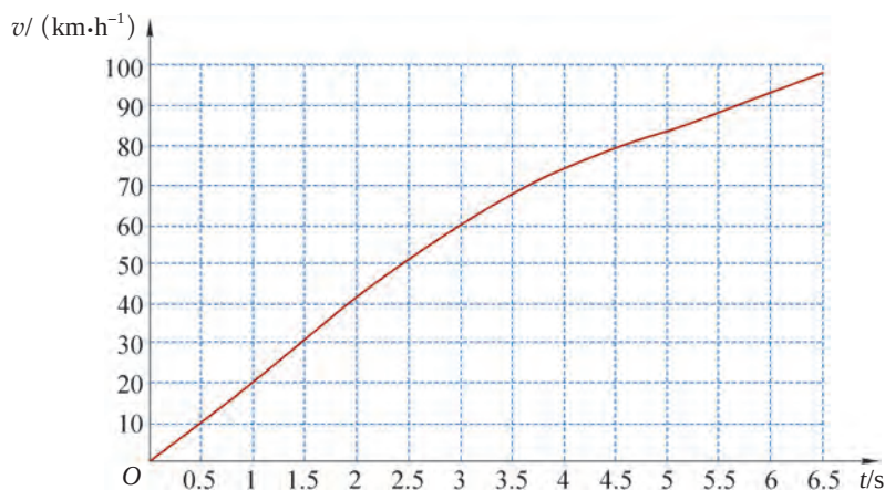
图 1-29 某品牌汽车 0~100 km/h 加速测试图示
