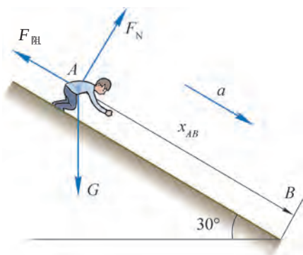
图4-32 运动员的受力分析
