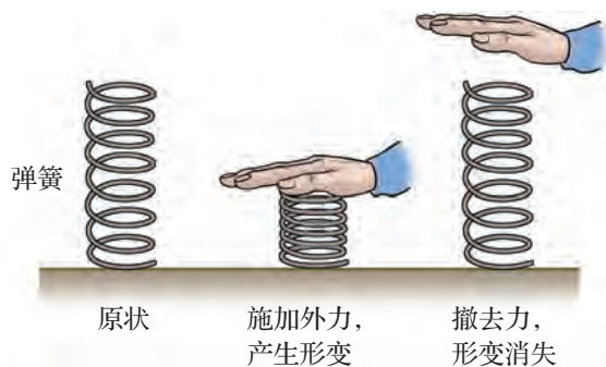
图 3-4 弹性形变
