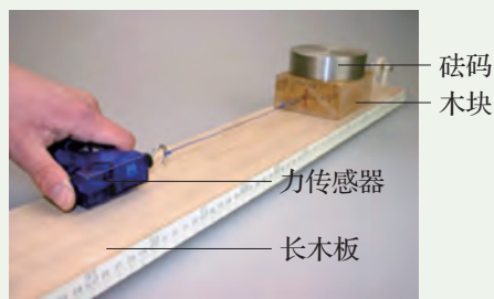
图 3-12 测量静摩擦力的大小
