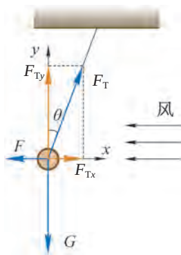
图 3-47 风力作用下小球的受力分析
