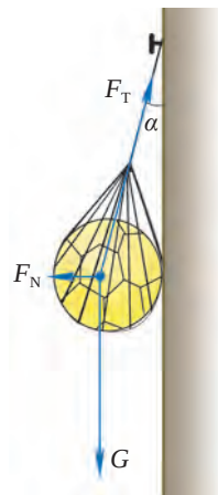
图 3-42 用网兜将球倚挂在墙上
