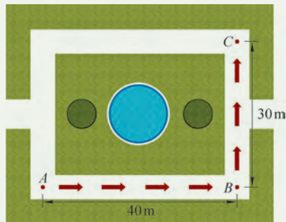
图 1-7 某同学的行走路径
