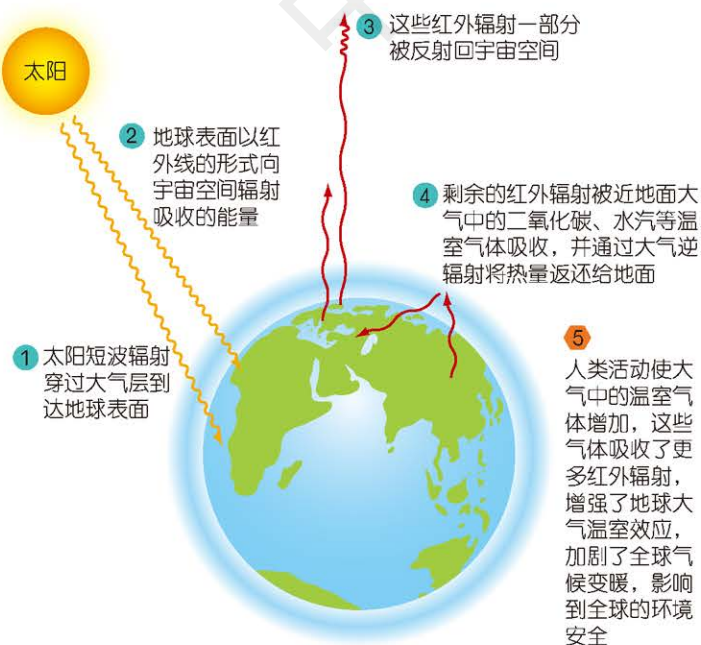
地球大气温室效应示意
