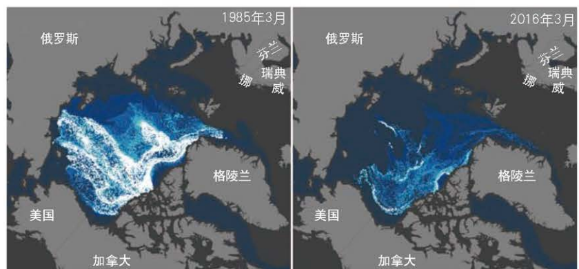
北冰洋冬季冰面最大时海冰年龄影像对比
