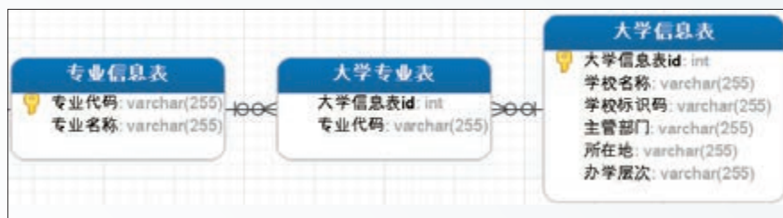
图3.3.7 表的关联
