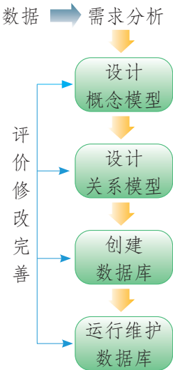
图3.1.2 大体过程
