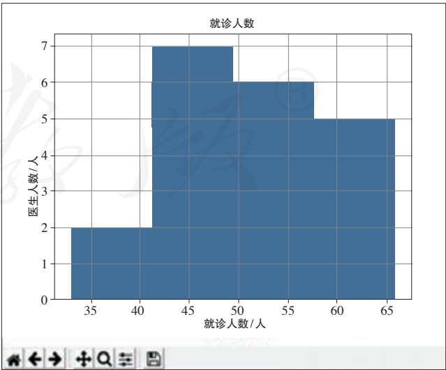
图4.1.4 直方图
