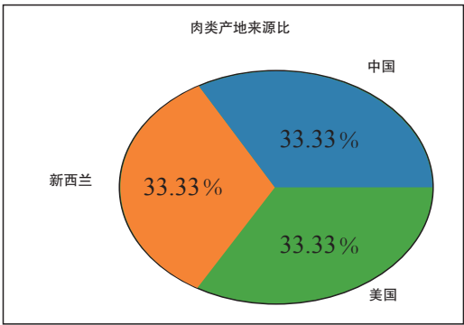
图 4.1.6 饼图
