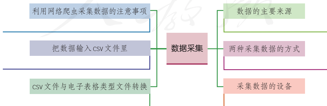
图2.2.13 知识总结
