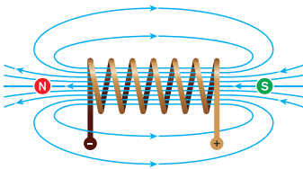
图2.3.3 干扰的出现
