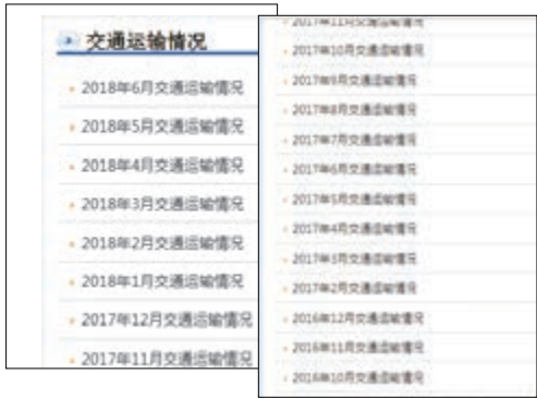
图 2.2.6 网页条目
