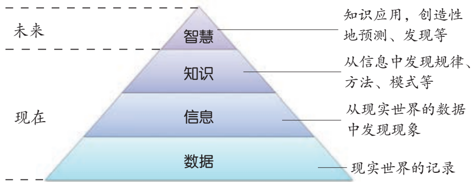
图 1.1.3 DIKW 金字塔
