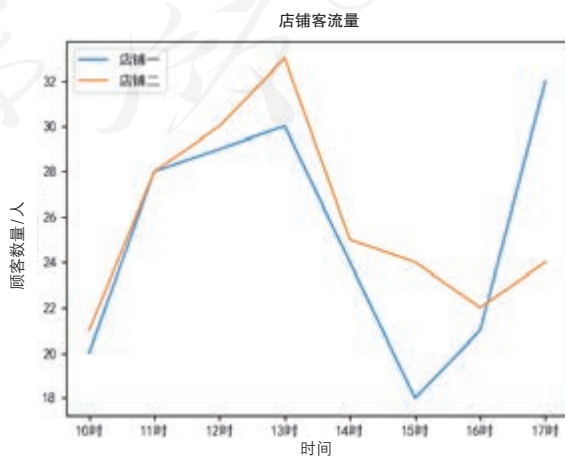
图4.1.2 对比分析图
