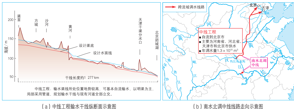
图 3.1.2 南水北调中线工程示意
