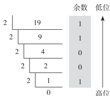
图1.2.7 除2反向取余法
