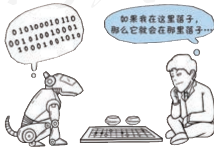
图4.1.1 人机博弈
