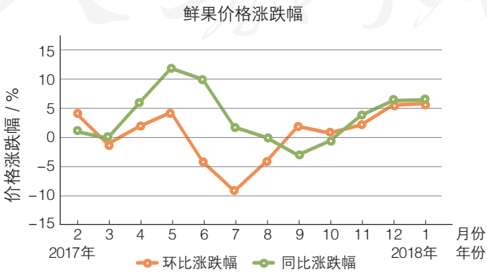
图 3.3.17 折线图示例
