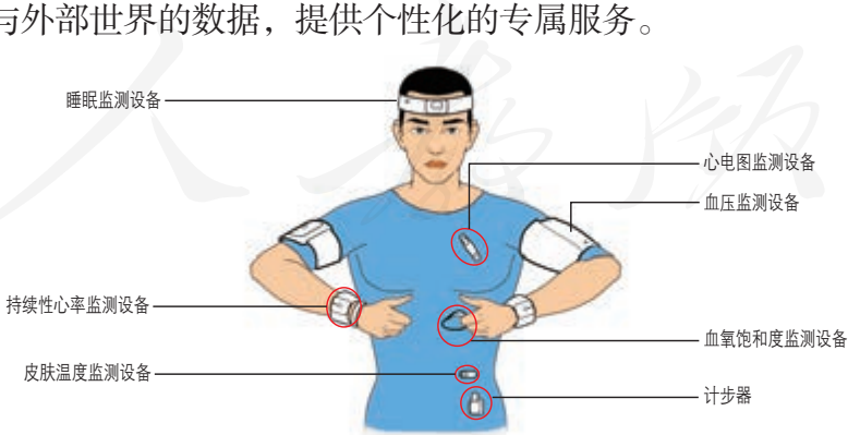
图 1.1.3 可穿戴设备
