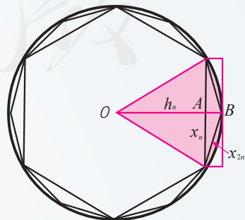
图2.4.3 “割圆术”示意图
