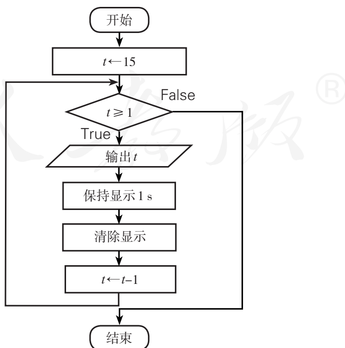
图 2.2.3 “倒计时 15 s” 算法流程图
