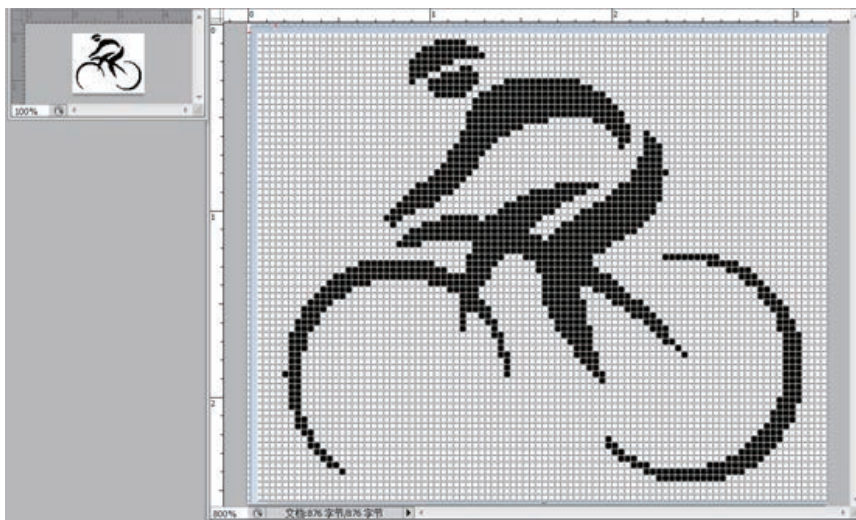
图 1.2.9 图像与像素
