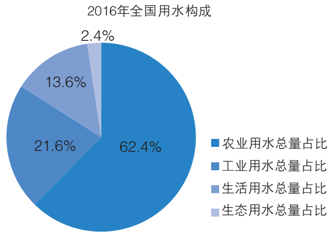
图 3.3.19 饼图示例
