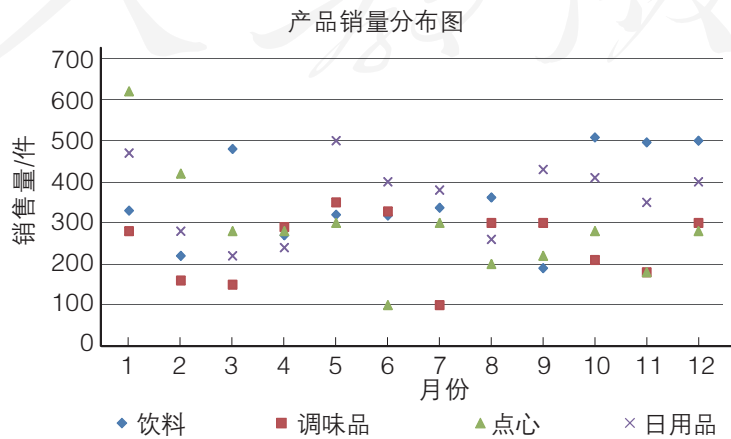
图 3.3.20 散点图示例
