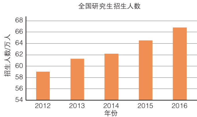
图 3.3.18 柱形图示例
