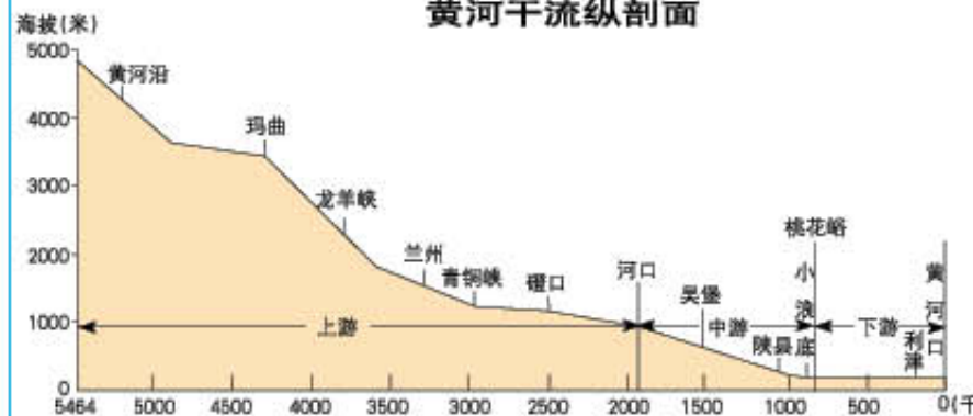
黄河干流纵剖面
